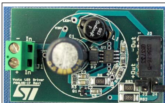
STEVAL-ILL007V1
